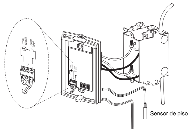
Conexiones para el sensor de red y de exterior (referirse a las secciones 7.2)
